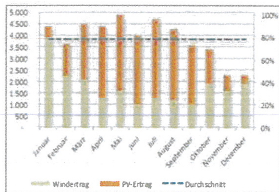
Verstetigung Stromertrag
